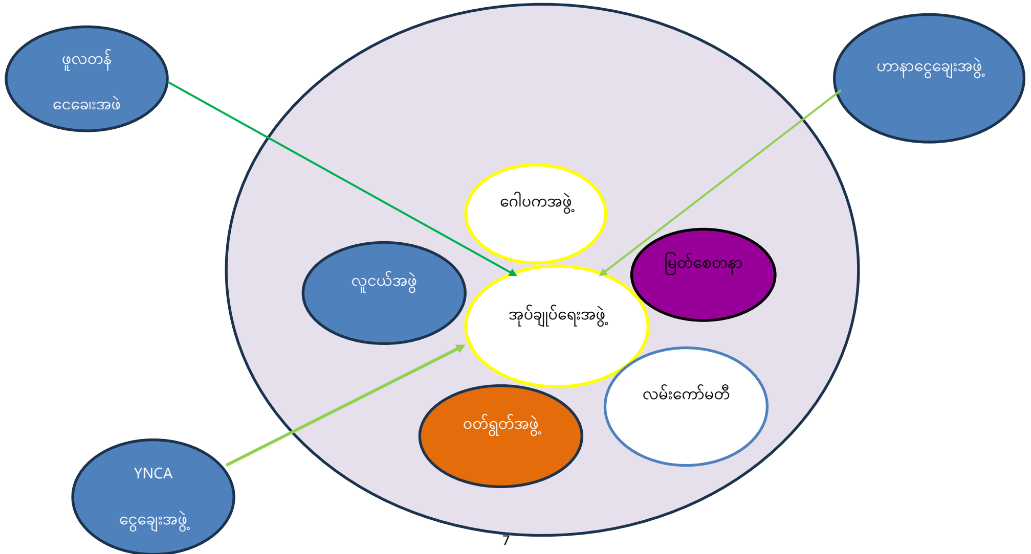
Venn Diagram
